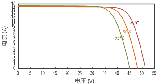
JT570SSt(B) 不同温度下的IV曲线
